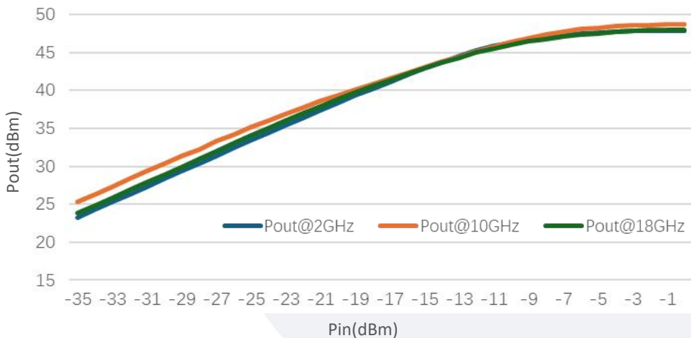
Pout@Pin
