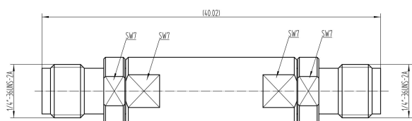
TLLF-DC-16G-FF
