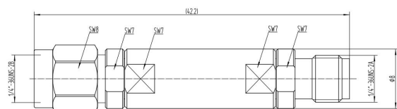
TLLF-DC-16G-K
