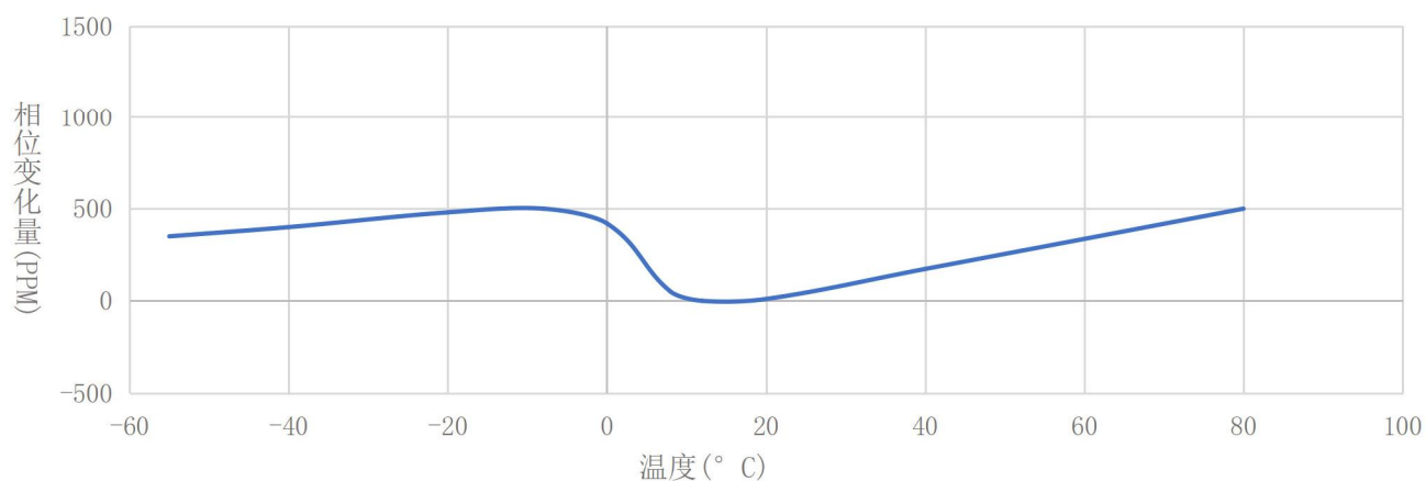
温度相位稳定性 (PPM)
