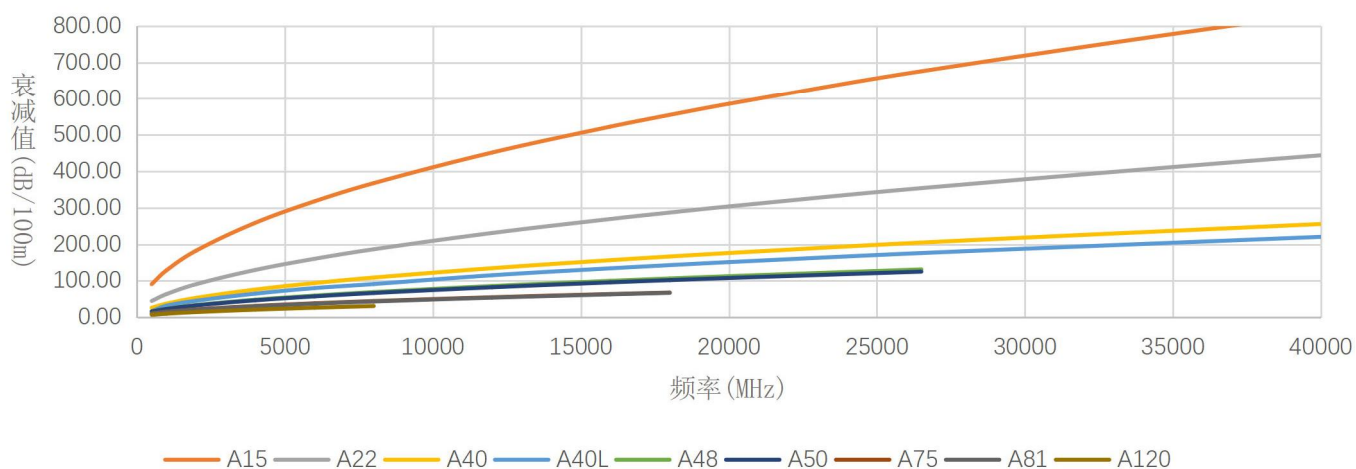
衰减VS频率
