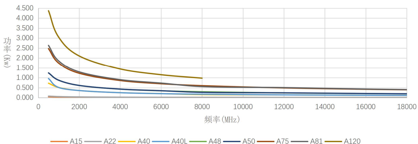
功率VS频率
