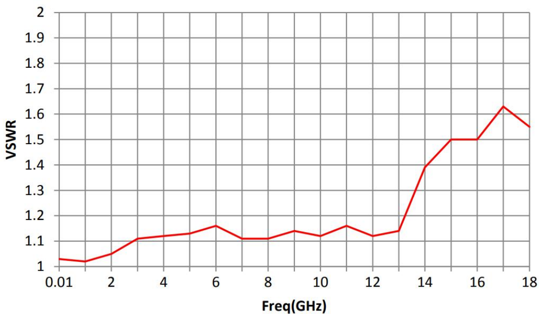
驻波比 VS 频率
