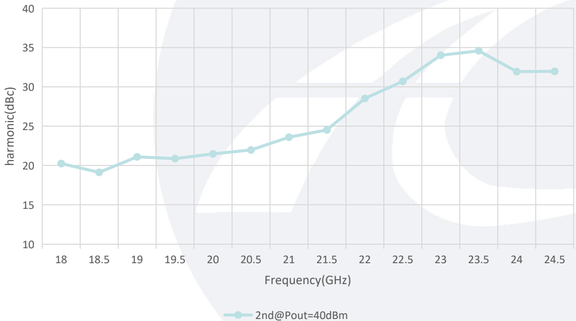
Harmonic@Pout=40dBm
