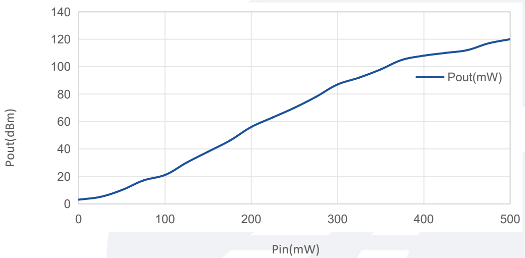
Output Power@Pin
