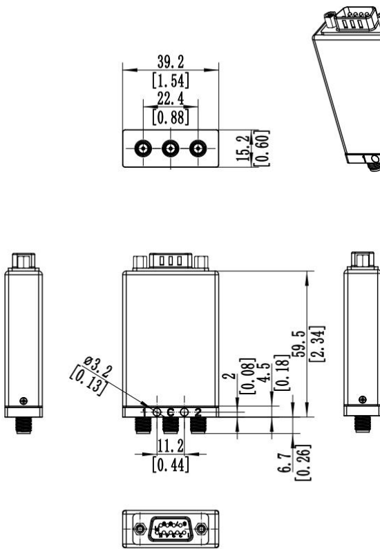
9 PIN 公头DSUB
