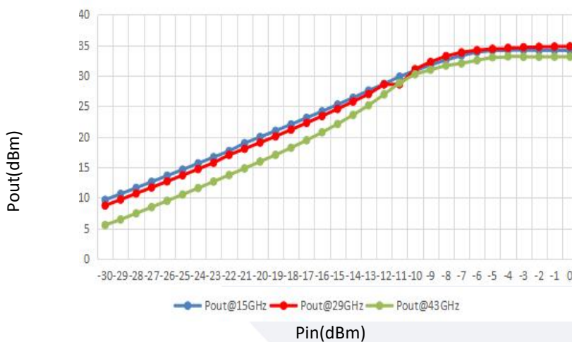
Pout@Pin
