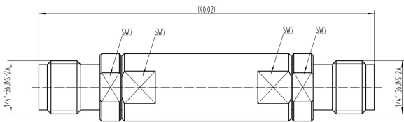
TLME-10G15G-5-FF
