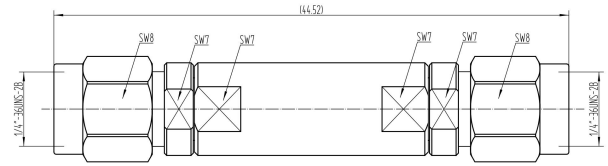
TLME-10G15G-5-MM
