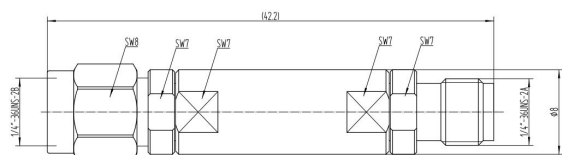
TLLF-DC-19G-K
